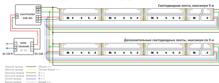
Схема 2. Подключение нескольких светодиодных лент с двух сторон
