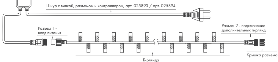
Рисунок 1. Схемы подключения.
