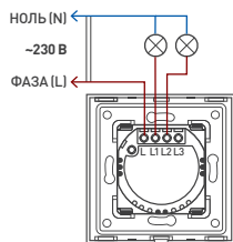
Рис. 2. Схема подключения (050041, 050038, 050039, 050040)
