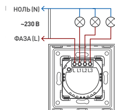
Рис. 3. Схема подключения (050042, 050048, 050047, 050046)
