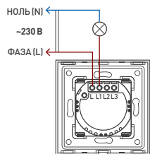
Рис. 1. Схема подключения (050035, 050037, 050036, 050033)
